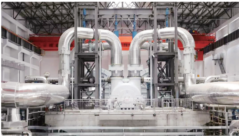
■肥城300MW先进压缩空气储能国家示范电站主厂房。(资料图) 通讯员供图
